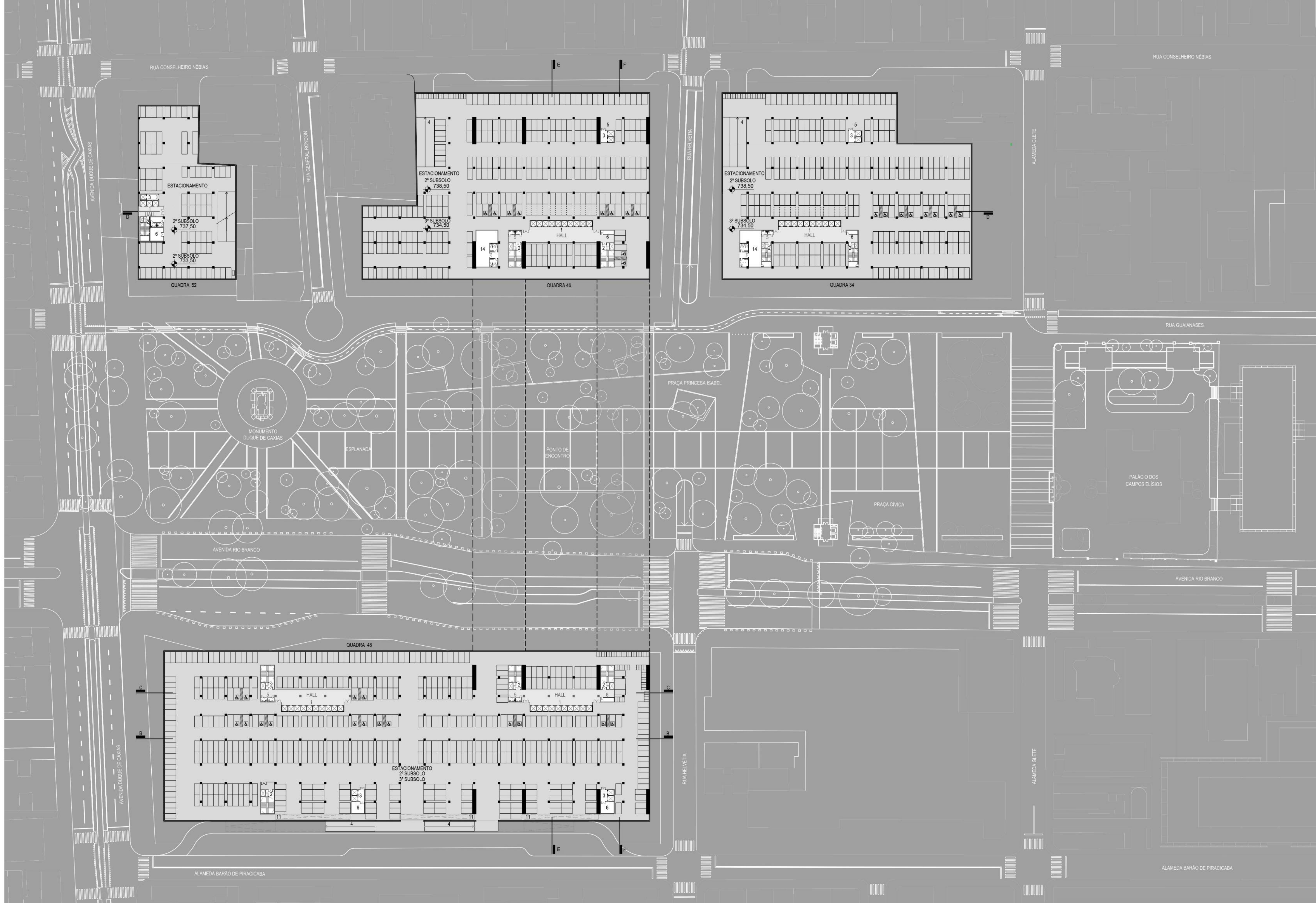
IMPLANTAÇÃO 2º / 3º SUBSOLOS - ESTACIONAMENTOS escala 1:750
