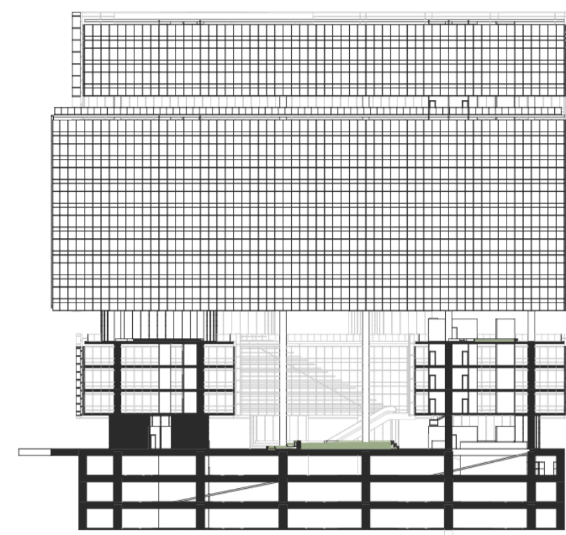
Corte C_esc 1/750
