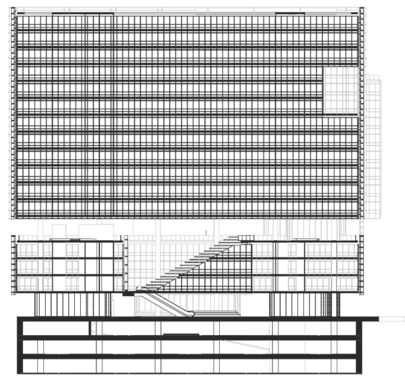
Corte B_esc 1/750
