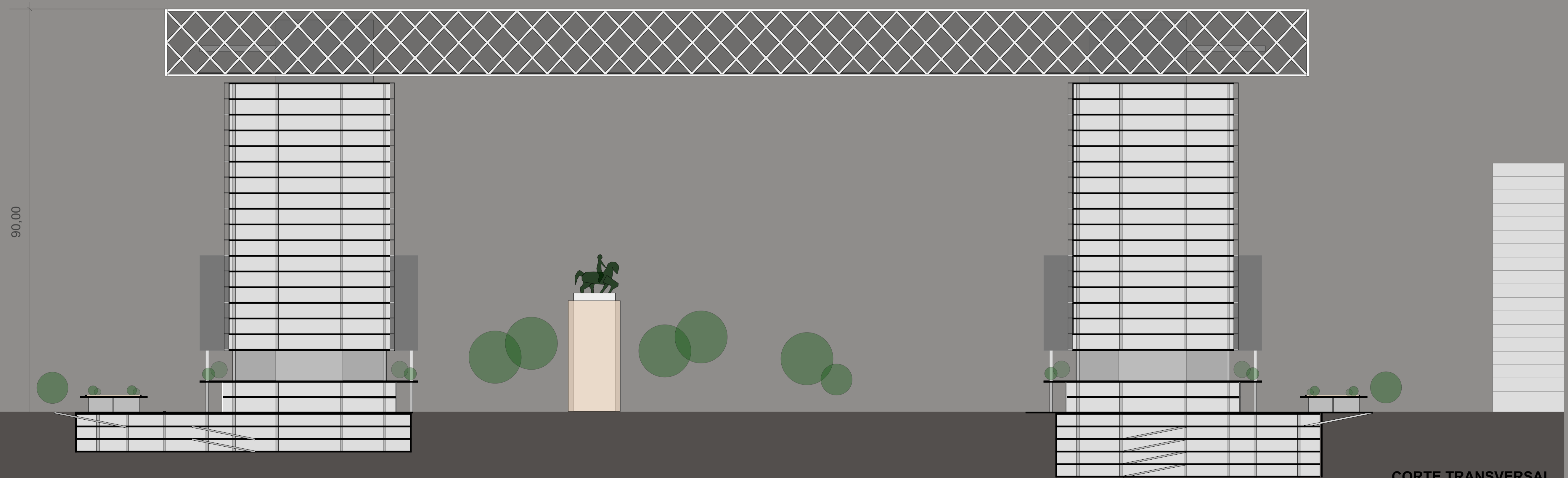
CORTE TRANSVERSAL ESC 1.500
