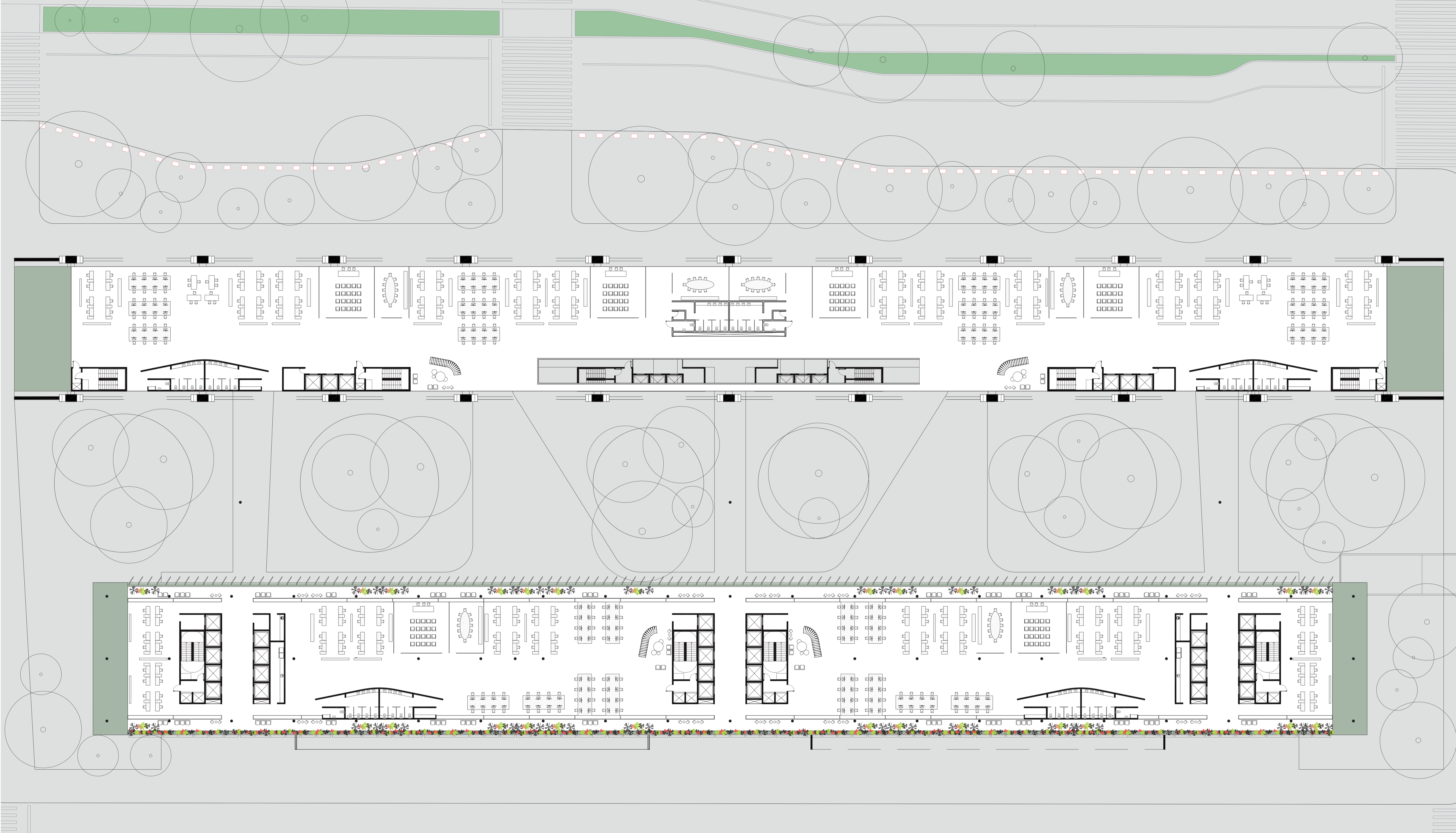
andar padrão administrativo do edifício longitudinal (1 ao 5 andar) e da torre (1 ao 20 andar) da quadra 48 1:250
